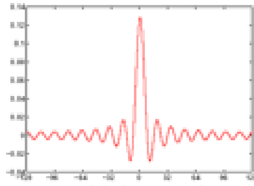
\text{sinc}(at)
